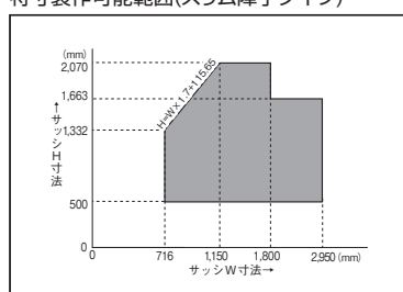
特寸製作可能範囲(スリム障子タイプ)
