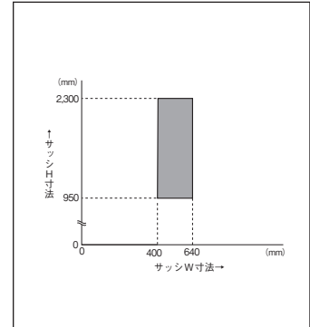
特寸製作可能範囲
