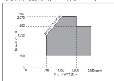
特寸製作可能範囲(スリム障子タイプ)
