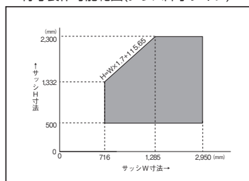
特寸製作可能範囲(テラス障子タイプ)
