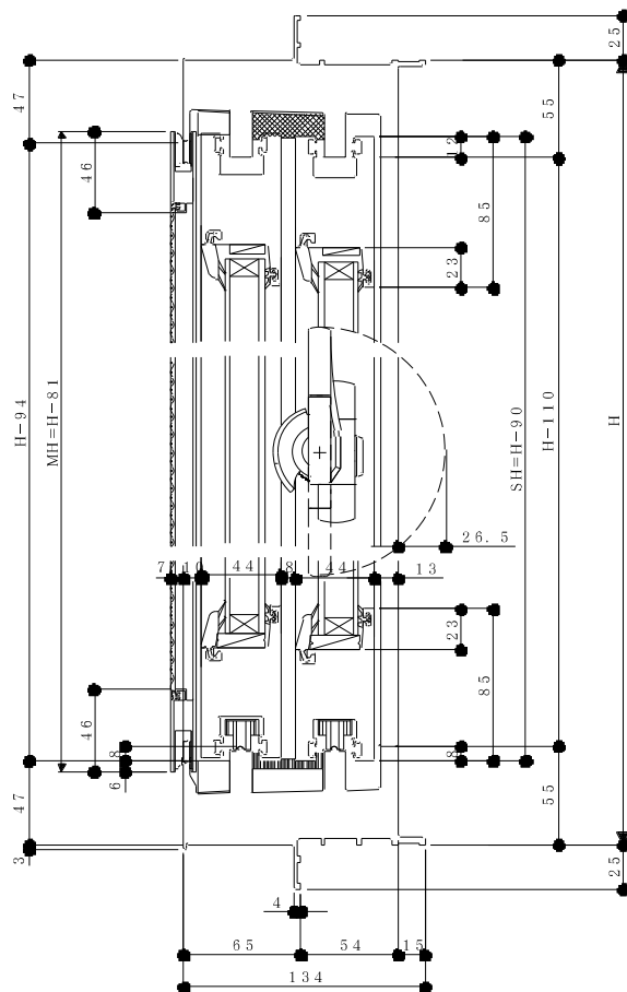
□縦断面図
