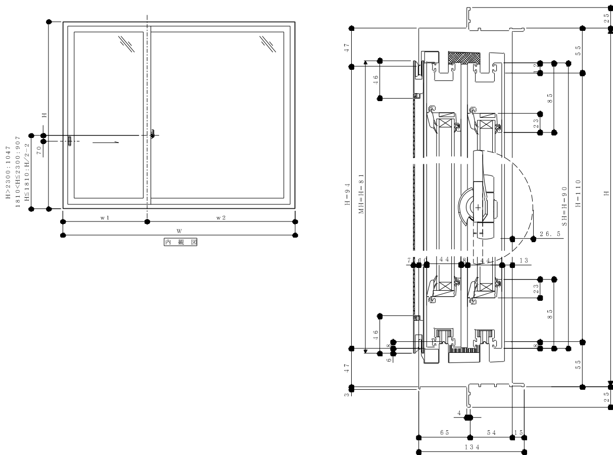
□縦断面図
