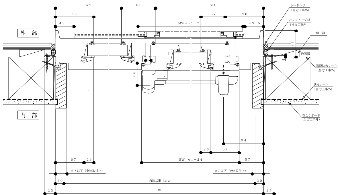
横断面図
