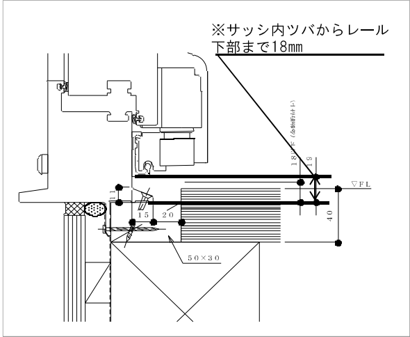
(下枠詳細寸法)
