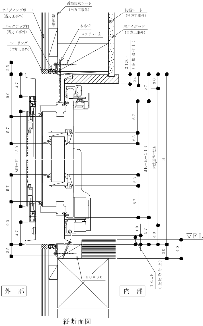
□縦断面図
