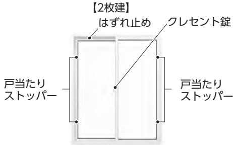
引違い窓
