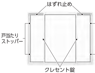
【両袖】
